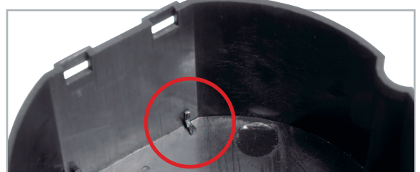
Bild 4: Modifikation der Unterputzdose: Die gekennzeichnete Gehäusenase ist wie hier gezeigt abzuschneiden.
