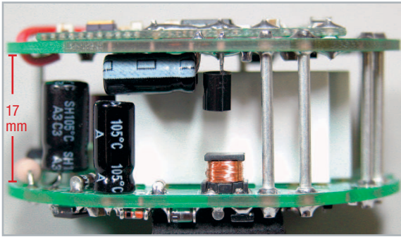
Bild 2: Detailaufnahme des Aufbaus. Der Elko C 109 ist liegend zwischen den Platinen montiert und es ist ein Abstand von 17 mm zwischen den Platinen herzustellen.
